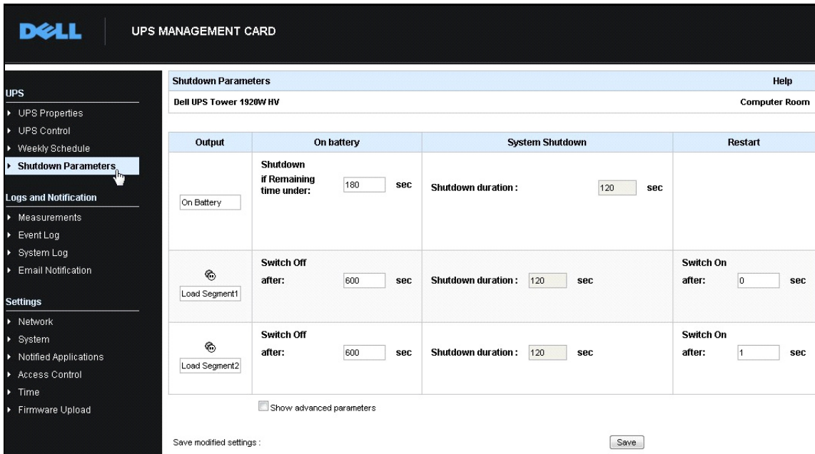
図 88.Dell ネットワーク管理カードウェブインターフェース
